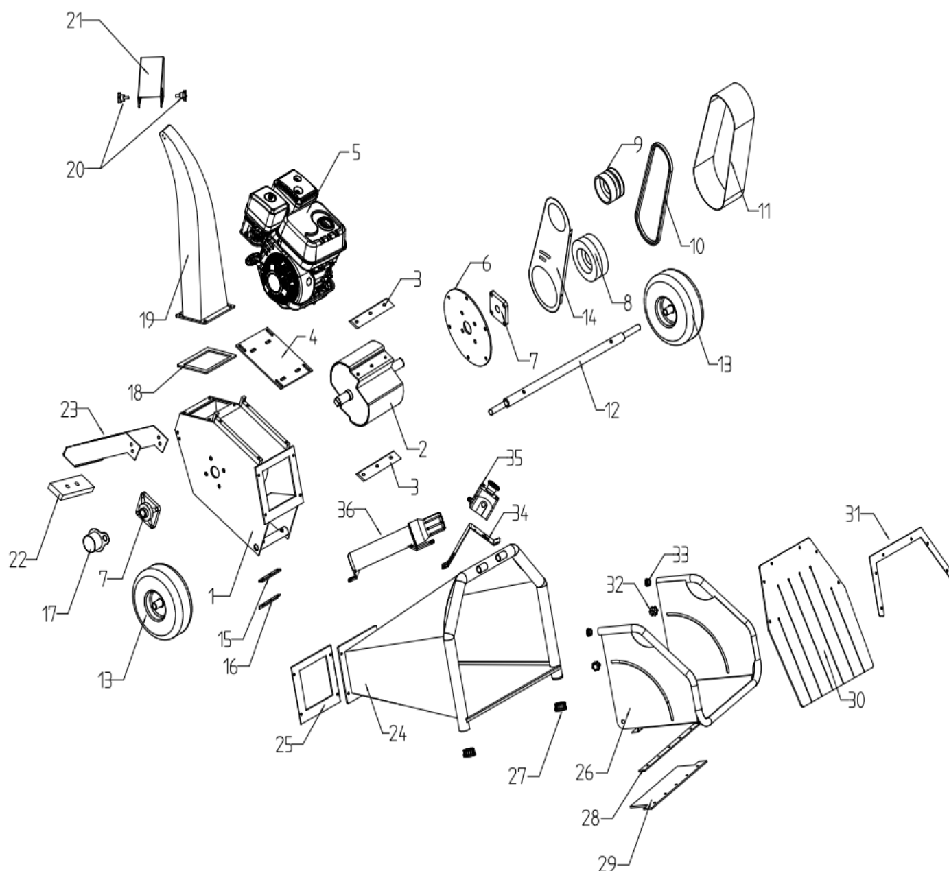
Rys. 1. Widok rozstrzelony — rozdrabniacz spalinowy KWCH302A
